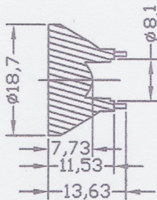
SECA-A
